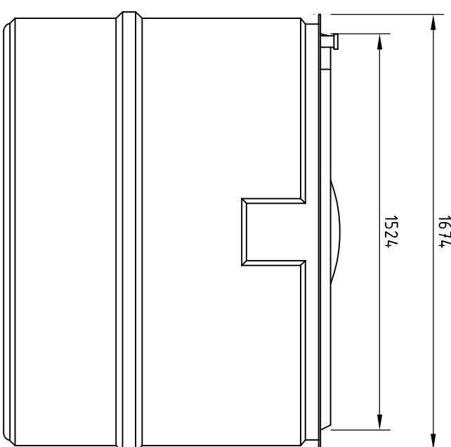
END ELEVATION
