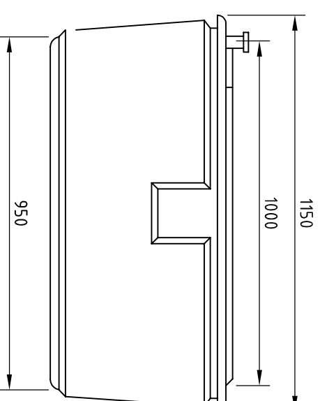
END ELEVATION
