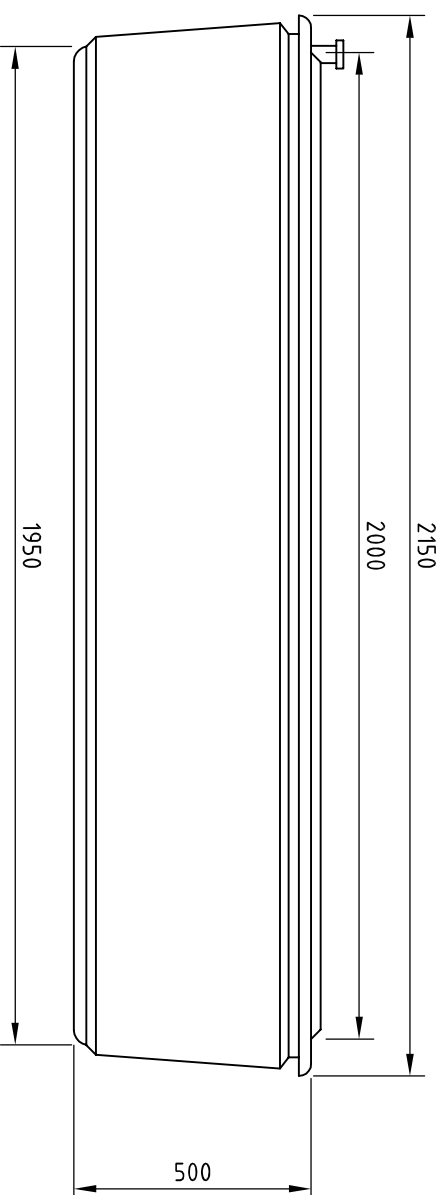
ELEVATION
