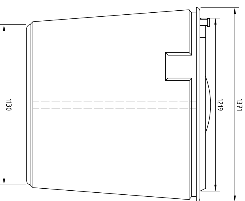
END ELEVATION
