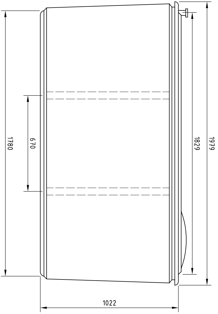
ELEVATION
