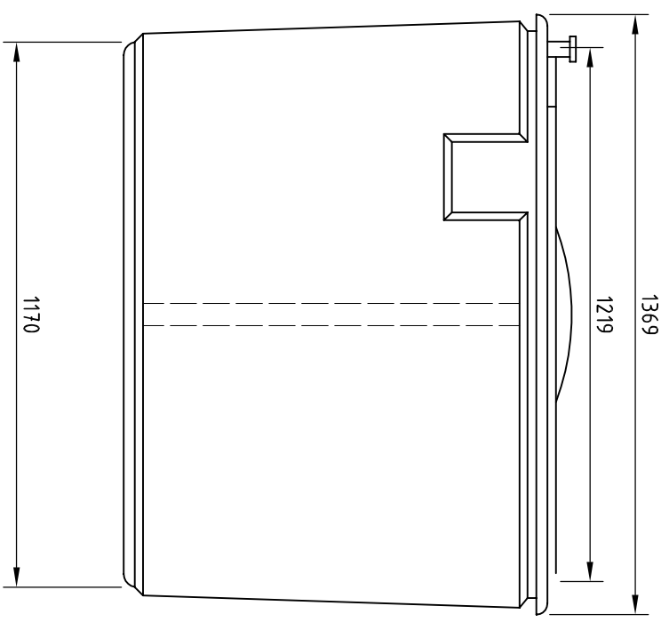
END ELEVATION
